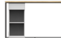
07 B 10.2/12 avec desserte, 1 tiroir et 1 tablette with cabinet, 1 drawer and 1 shelf 1200 x 760 x 550 mm M2/20.42.12.02 1.251,00 €
